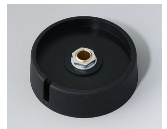
A3050069 COM-KNOBS 50, avec un évidement PA 6 néro 50x16mm 6mm
