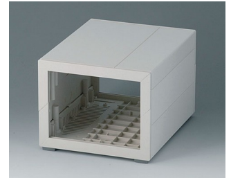
B2213217 MEDITEC E 160, sans poignée étrier ABS (UL 94 HB) gris blanc RAL 9002 160x200x124mm IP 40
